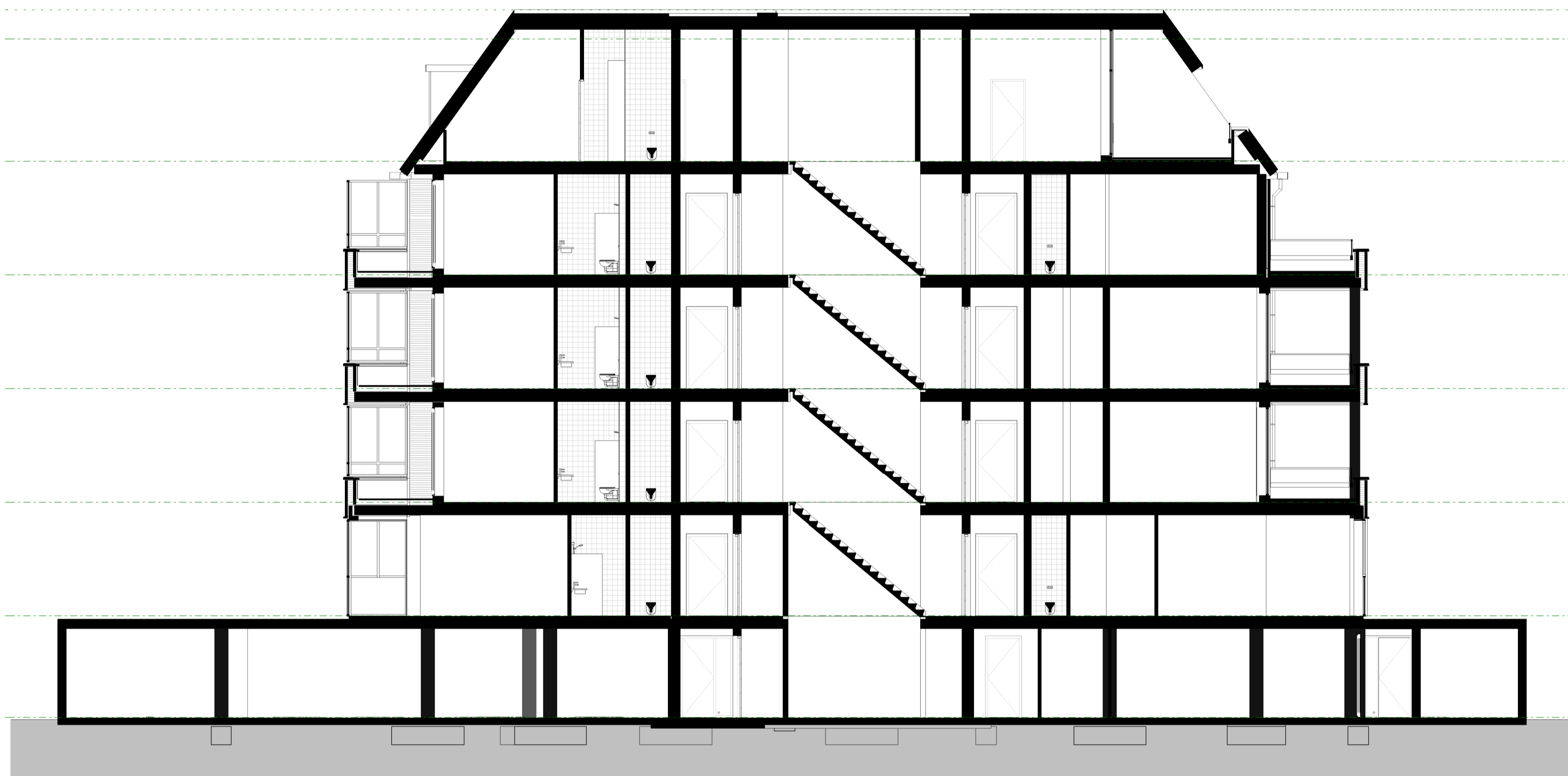
DOORSNEDE A-A
