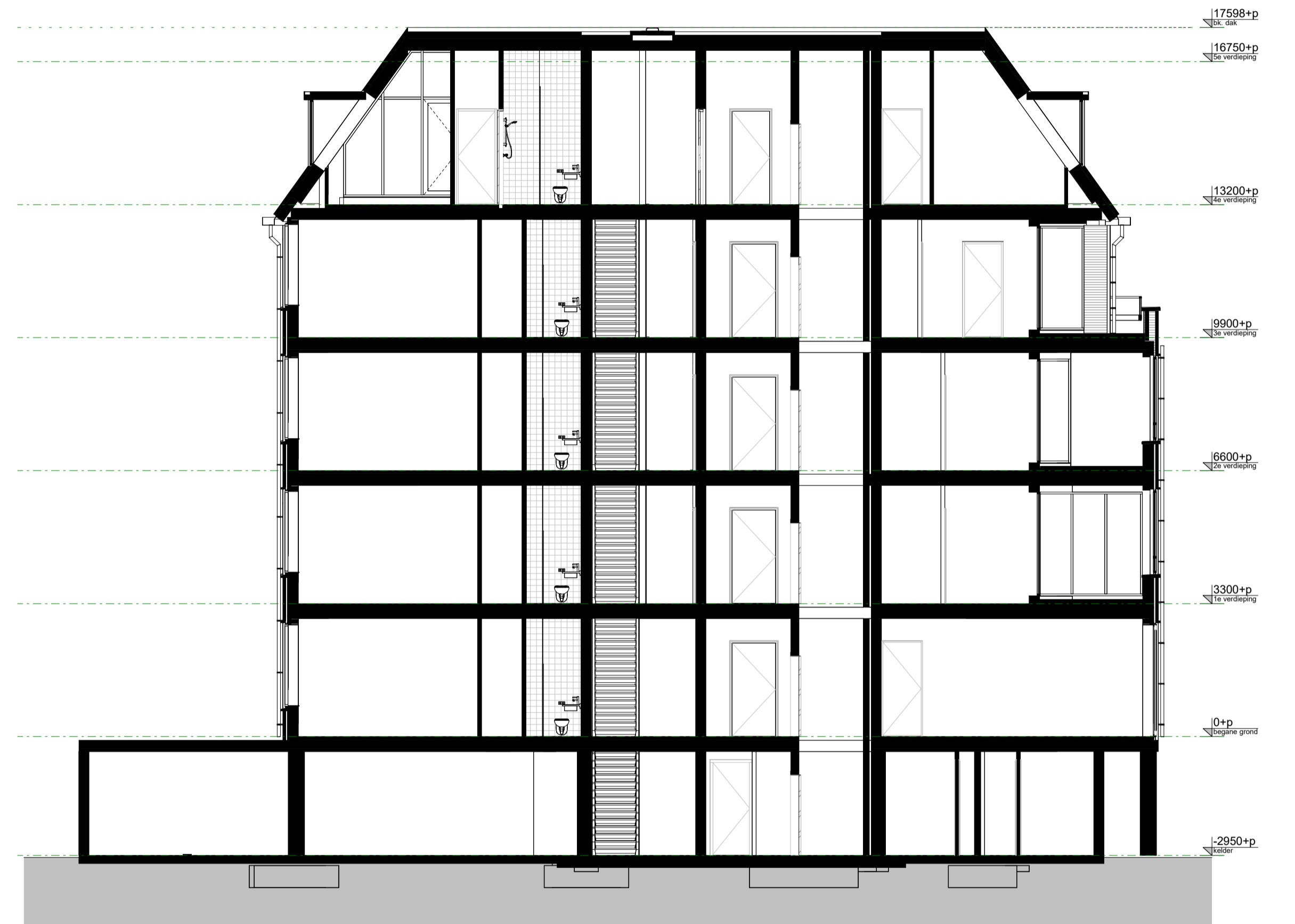
DOORSNEDE B-B
